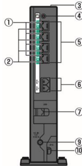
背面 PR-500XX/GE-ONU
