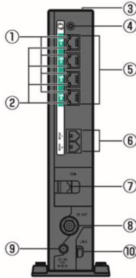
背面 PR-500XX/GV-ONU
