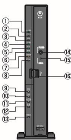
前面 PR-500XX/GV-ONU (①~②、⑭~⑯は、PR-500XX/ GE-ONU も同様) (①~⑩・⑭~⑯は、RT/RS も同様)
